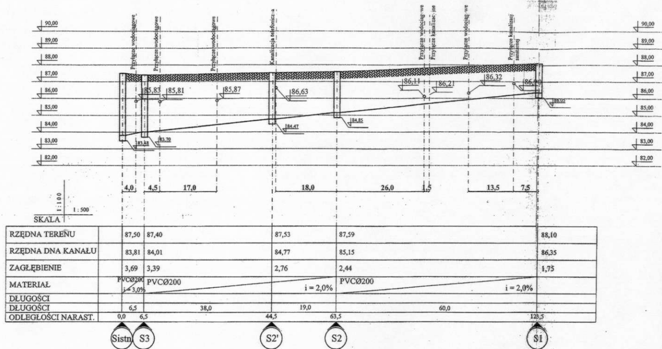
SIEĆ KANALIZACJI DESZCZOWEJ W UL. TADEUSZA KUTRZEBY L=123,5m, PVC Ø200
