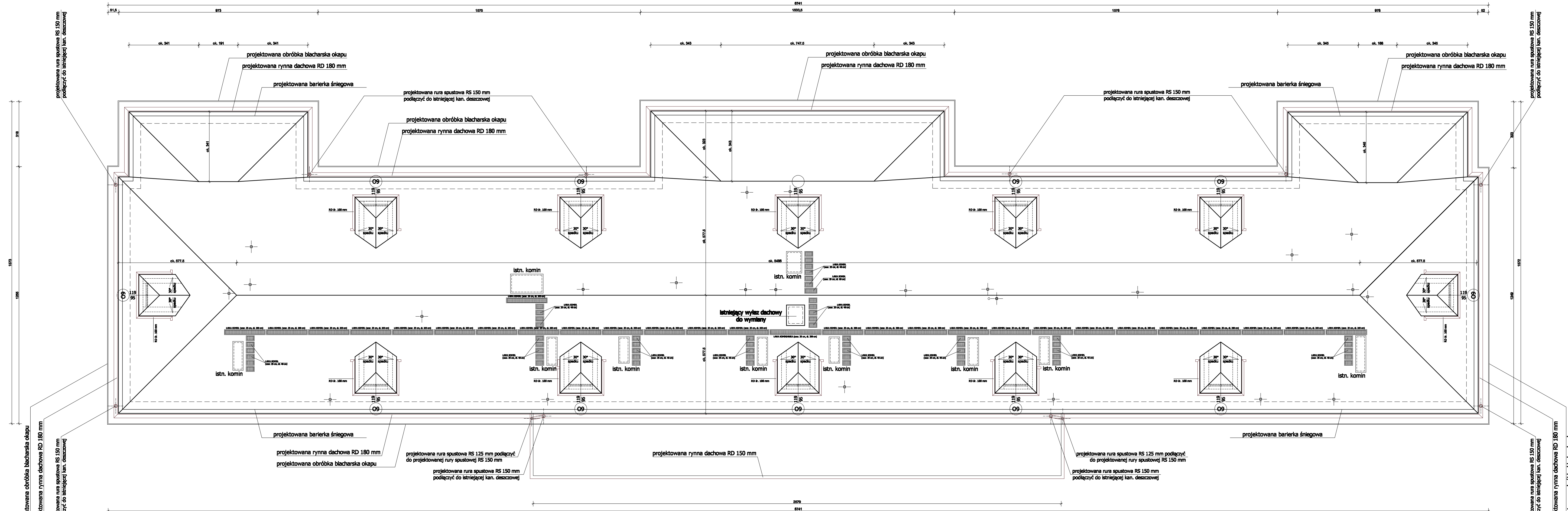
SCHEMAT UKŁADU POŁĄCZI DACHOWYCH - stan projektowany, skala 1:100
