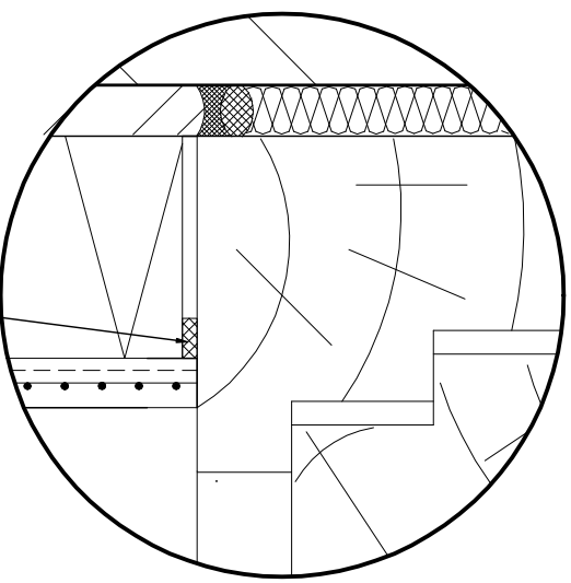
Szczegół A taśma uszczelniająca
