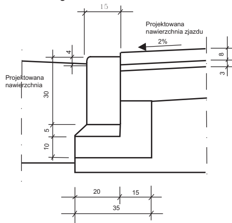
Szczegóły A
