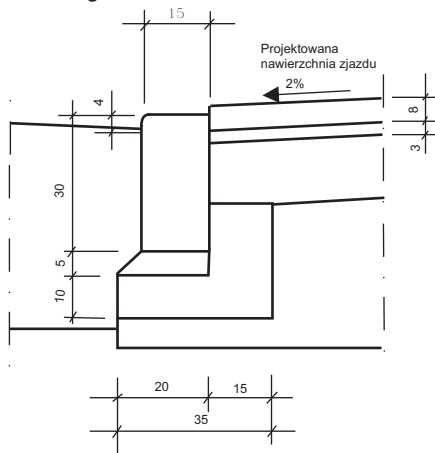
Szczegół A
